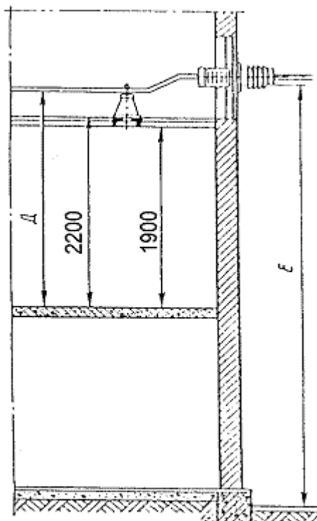
Фиг. 21. Минимални разстояния от неограничени тоководещи части и от долния ръб на изолаторите до пода; светла височина на коридора в ЗРУ; минимални разстояния от неограничени
