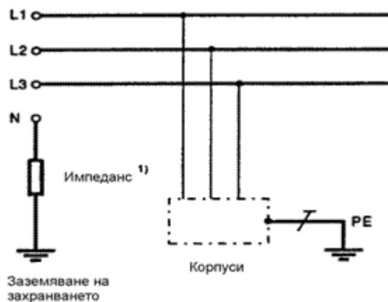
Фиг. 5. Схема IT
