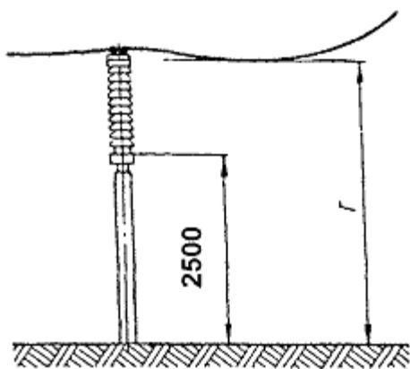
Фиг. 11. Минимални разстояния от неоградени тоководещи части и от долния ръб на изолаторите до земята.
