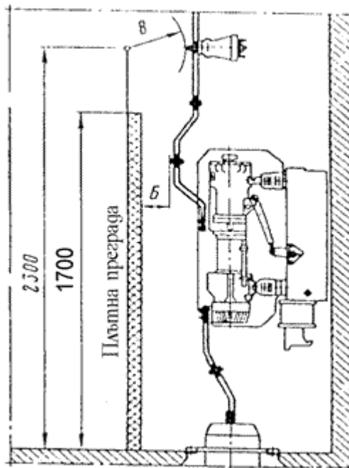
Фиг. 19. Минимални разстояния между тоководещи части и плътни огради
