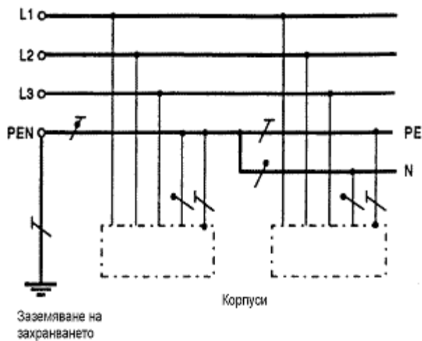
Фиг. 2. Схема TN-C-S
