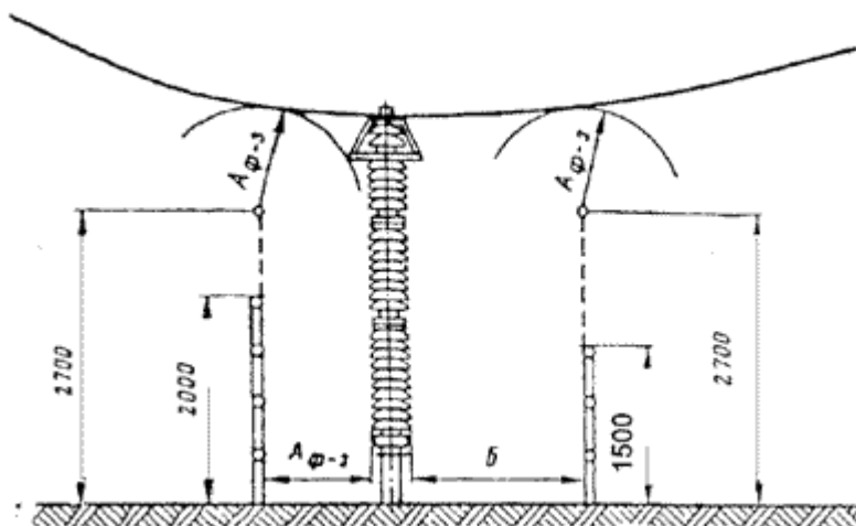
Фиг. 10. Минимални разстояния от тоководещи части и от елементи на изолатори, които се намират под напрежение, до постоянни вътрешни огради.
