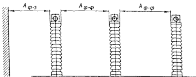
Фиг. 8. Минимални светли разстояния при твърди шини между тоководещи части и заземени части ( A_{\phi-з} ) и между тоководещи части на различни фази ( A_{\phi-\phi} ).
