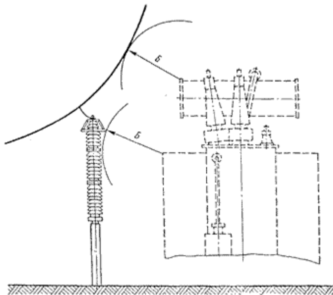
Фиг. 12. Минимални разстояния от тоководещи части до транспортни средства и до превозваните от тях съоръжения.
