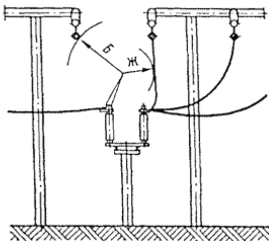
Фиг. 16. Минимални разстояния от контактите и ножовете на разединители в изключено положение до заземени и тоководещи части.
