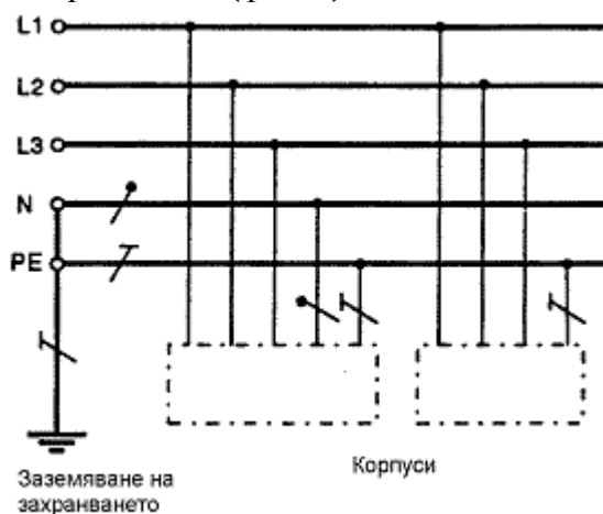
Фиг. 1. Схема TN-S
