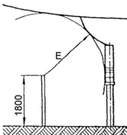
Фиг. 15. Минимални разстояния от тоководещи части до горния ръб на външна ограда.
