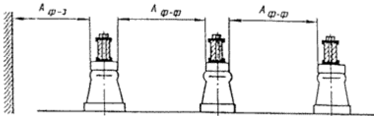
Фиг. 18. Минимални разстояния между тоководещи части на различни фази ( A_{\phi-\phi} ) и между тях и заземени части ( A_{\phi-З} )
