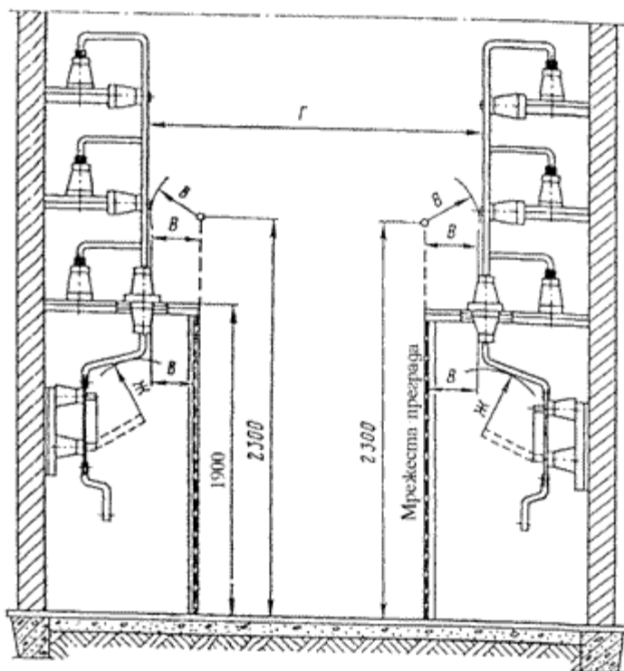
Фиг. 20. Минимални разстояния от тоководещи части до огради с мрежи и между неограничени тоководещи части на различни вериги
