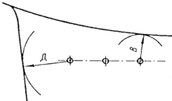
Фиг. 13. Минимални разстояния между тоководещи части на различни вериги, разположени в различни равнини, при обслужване на по-нискостоящата верига и наличие на напрежение на по-високостоящата верига.
