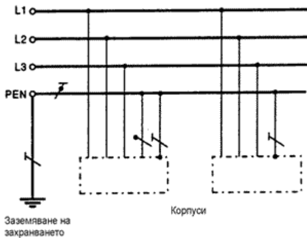
Фиг. 3. Схема TN-C
