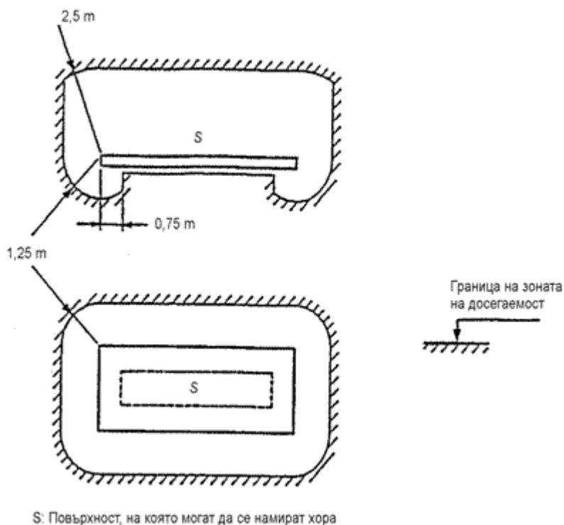
Фиг. 7. Зона на досегаемост при напрежения до 1000 V
