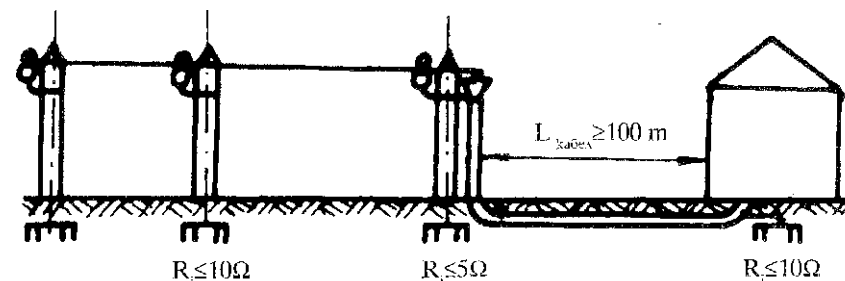
фиг.1 Схема за защита на склада за взривни материали от внасяне на високи потенциали чрез въздушни електропроводи.
