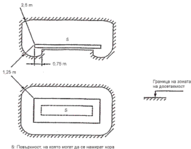
Фигура П1.1. Зона на досегаемост
