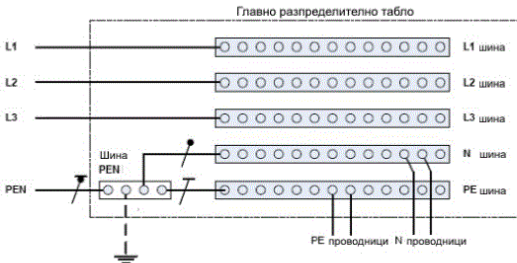
Фигура П7.1б. Пример 2 за свързване на PEN проводник.
